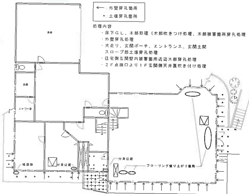
1階平面図
